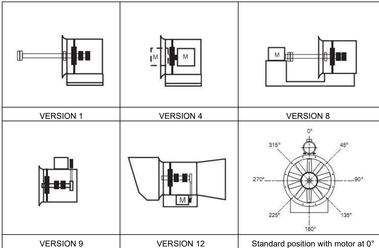
Fig. 2-1 Axial fan versions
